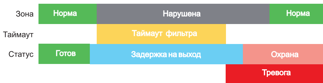
Рисунок 12. Превышен тайм-аут фильтра для зоны периметр во время задержки на выход
