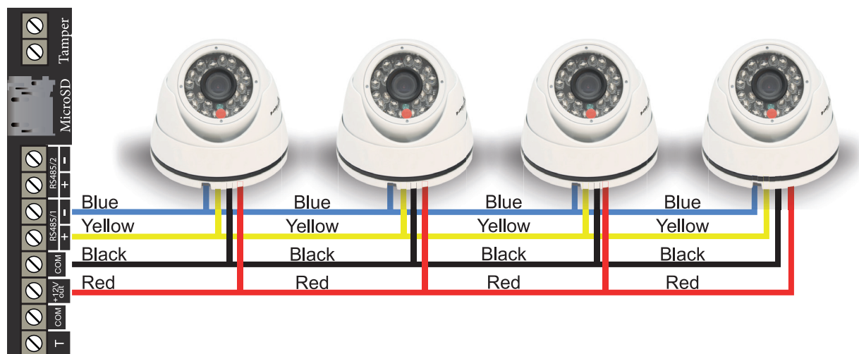
Рисунок 8. Подключение камер NV DOM 485-28IR к NV 2116
