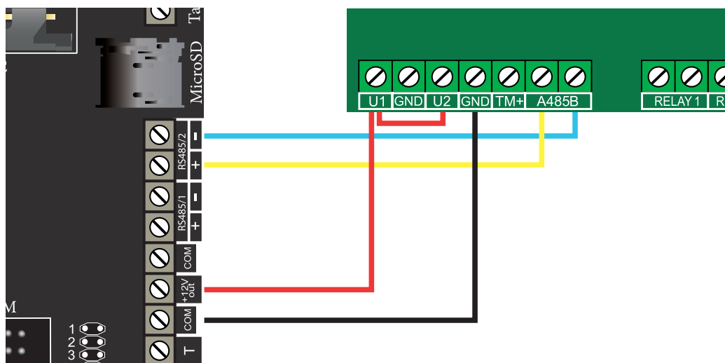
Рисунок 7. Подключение модуля Астра-РИ-М РР к NV 2116
