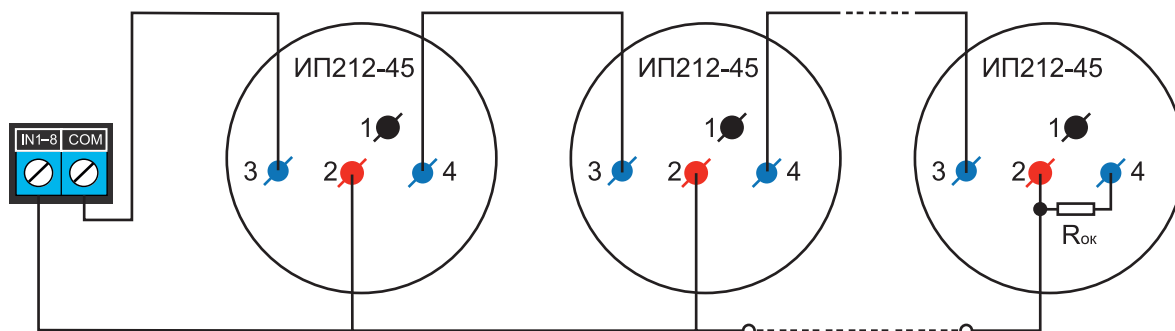
Рисунок 3. Схема подключения ИП212-45 к пожарному входу NV 2116 только с окончательным резистором
