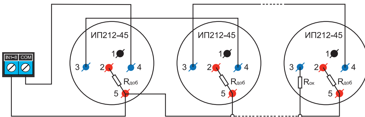
Рисунок 2. Схема подключения ИП212-45 к пожарному входу NV 2116 с добавочными и с оконечными резисторами
